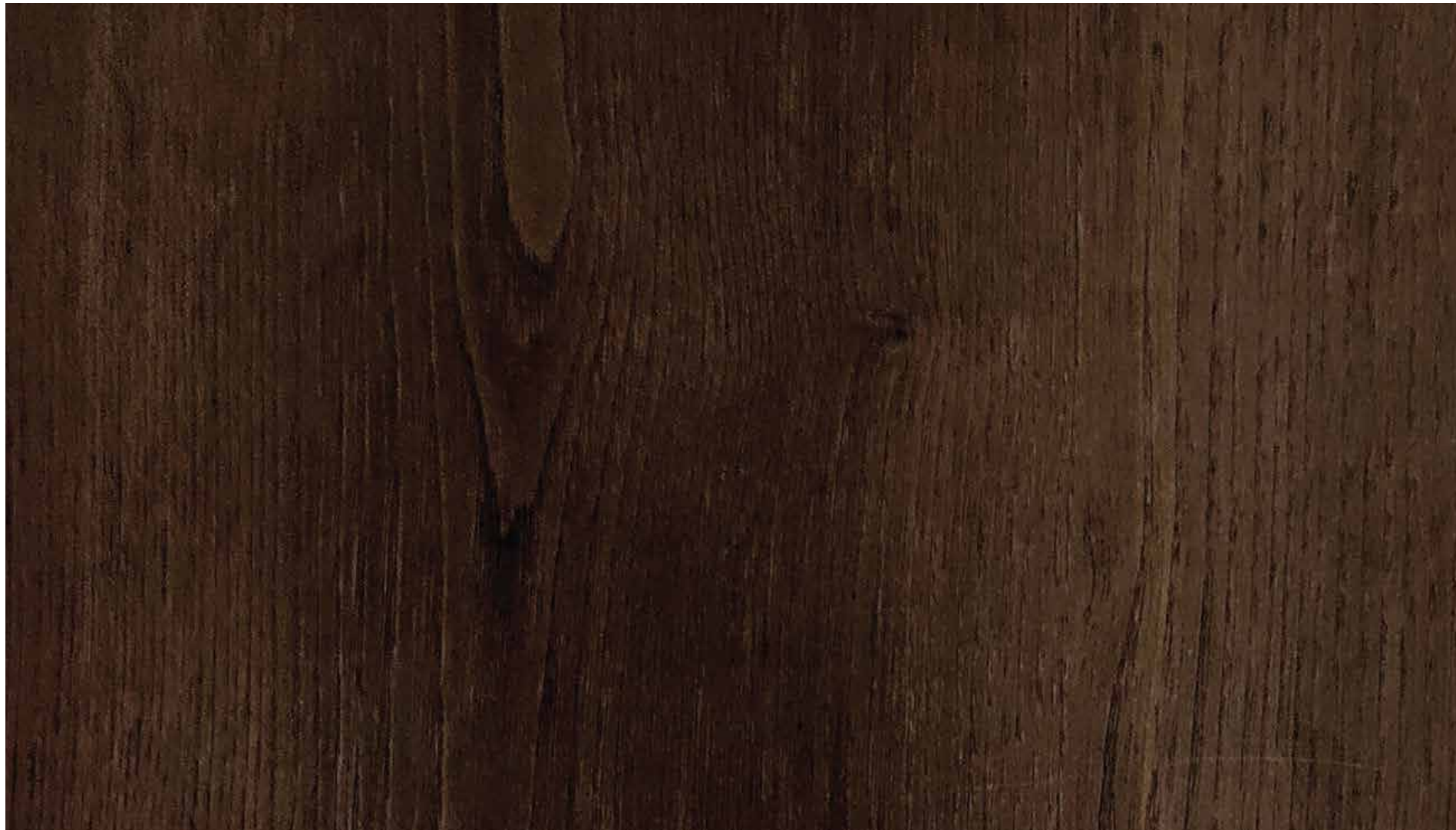
1039 KS | TANNED.OAK
