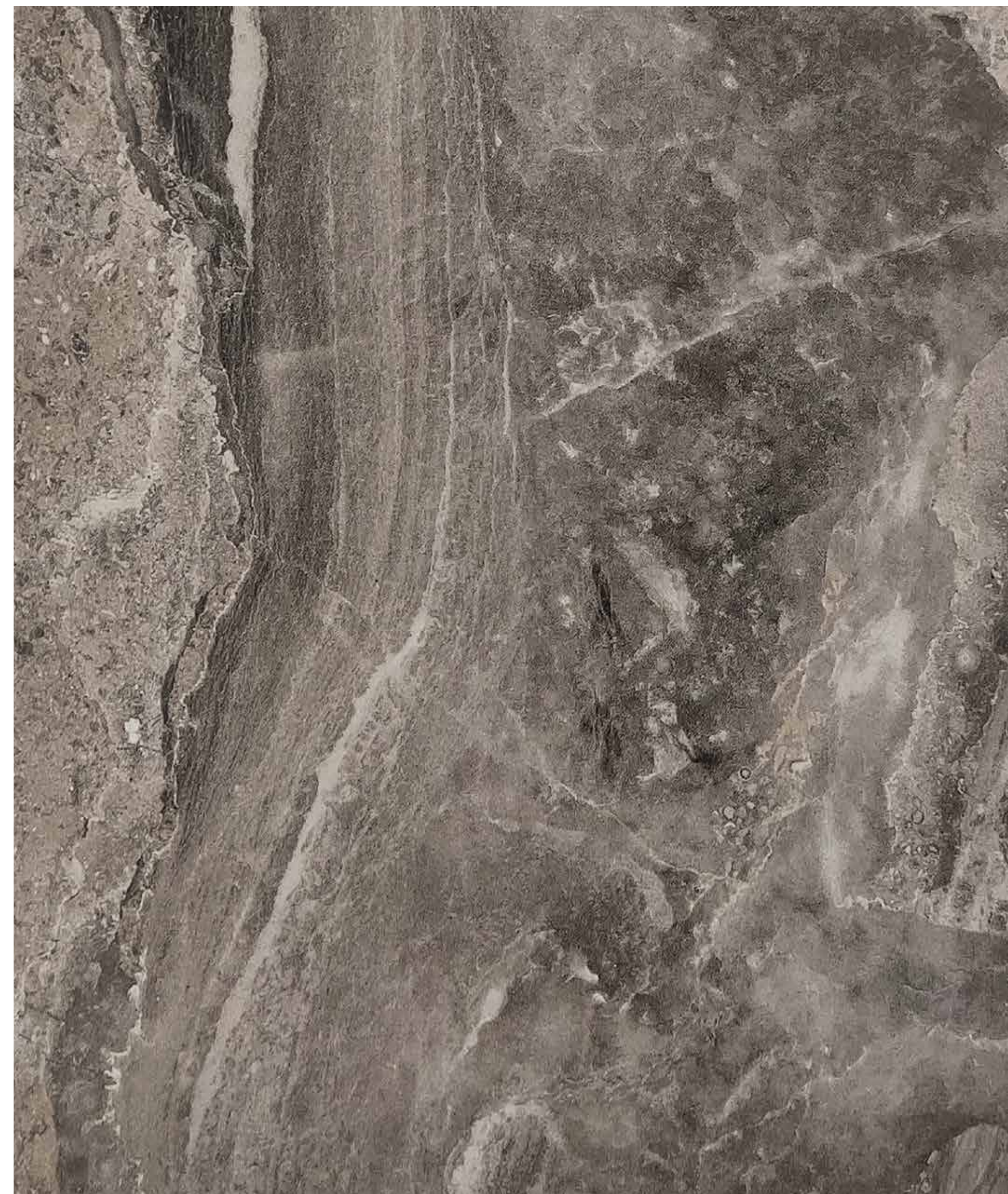
1502 SM | PALADINA
